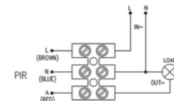
Схема подключения 25821 6, 25822 3, 25823 0, 25824 7, 25831 5, 25832 2, 25828 5, 25829 2
